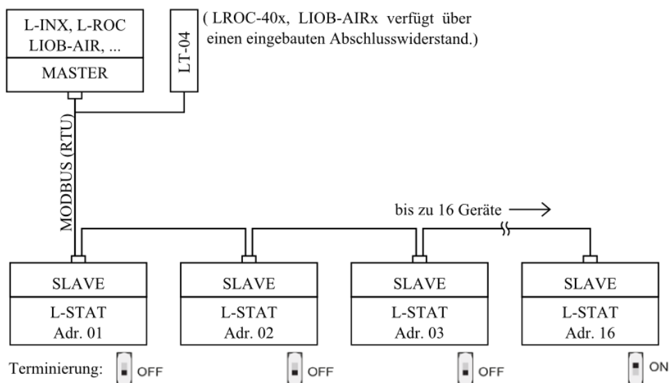
Abbildung 7: Modbus Netzwerk
