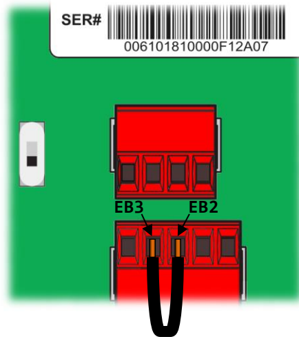
Abbildung 18: Kabelbrücke EB2-EB3
