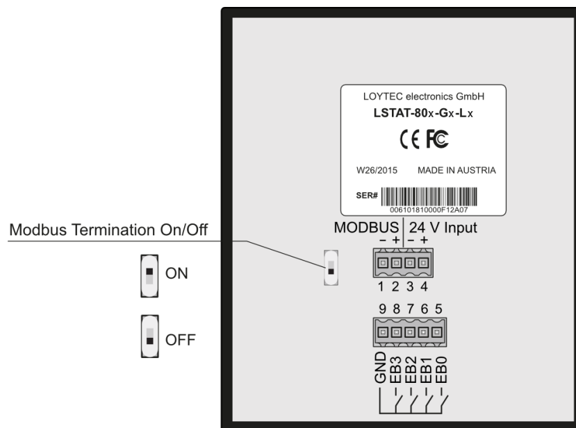
Abbildung 2: Rückansicht LSTAT-80x-Gx-Lx
