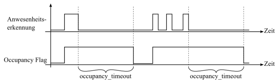
Abbildung 9: Bewegungsmelder Funktion
