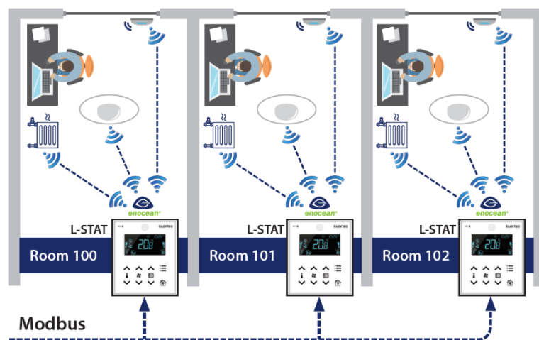
Abbildung 16: Beispiel Installationsschema
