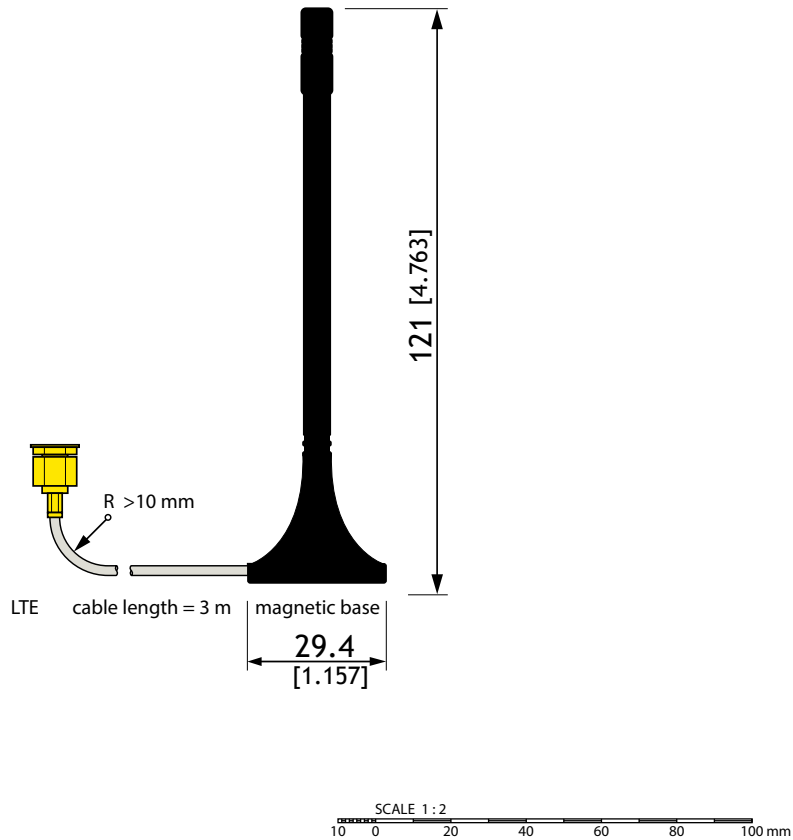
DIM060 LTE Antenna 700 - 2600 MHz
